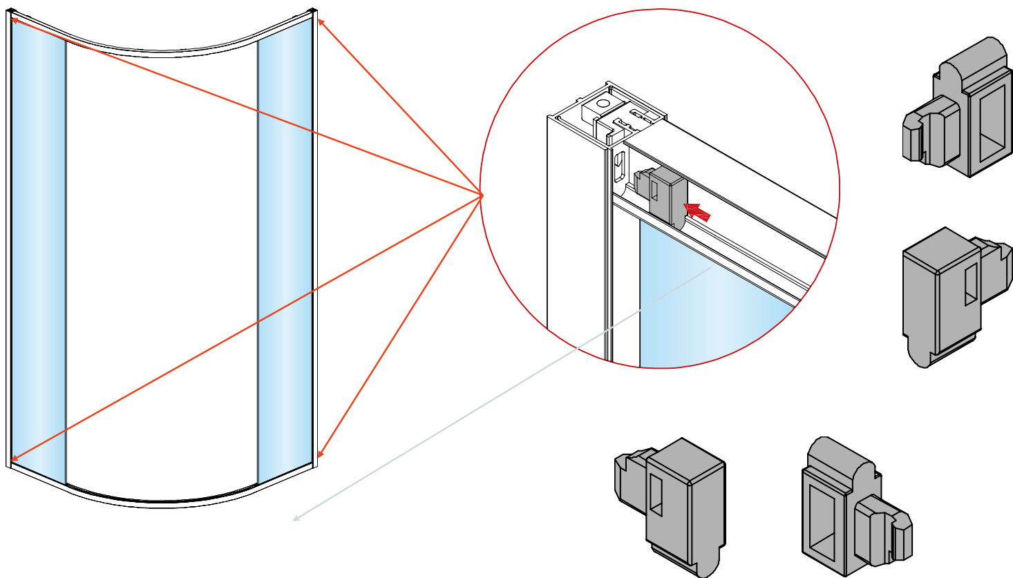
INSERIRE IL PEZZO INDICATO NEL PROFILO VERTICALE IN MODO DA BLOCCARE IL MONTAGGIO TRA IL PROFILO ORIZZONTALE E QUELLO VERTICALE.
