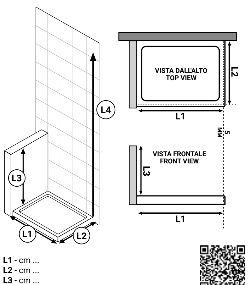
"L" - Spazio in angolo con muretto Sx Corner shower enclosure with half wall on the left. Eckdusche mit niedriger Mauer links. Cabine de douche d'angle avec muret bas à gauche.
