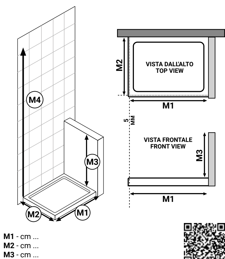
"M" - Spazio in angolo con muretto Dx Corner shower enclosure with half wall on the right. Eckdusche mit niedriger Mauer rechts. Cabine de douche d'angle avec muret bas à droite.
