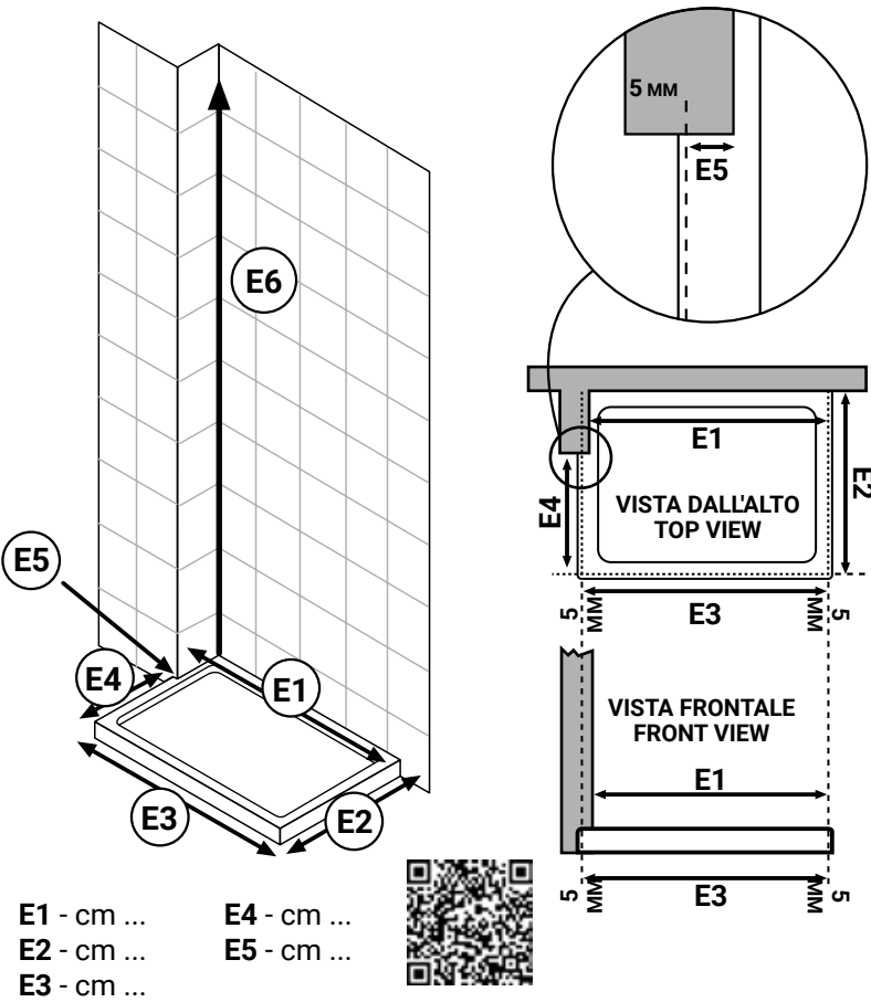
"G" - Spazio in nicchia con muretto Sx Niche with half wall on the left. - Nische mit niedriger Mauer links. Niche avec muret bas à gauche.
