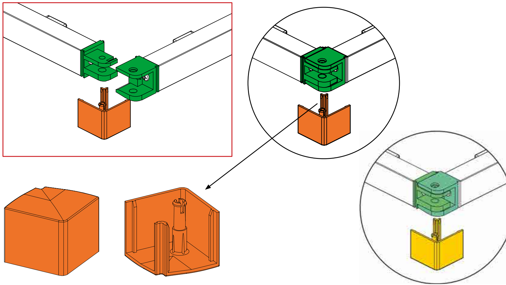
UNIRE I DUE PROFILI ORIZZONTALI COME INDICATO IN DISEGNO E POI CHIUDERE IL TUTTO CON IL CORNER.
