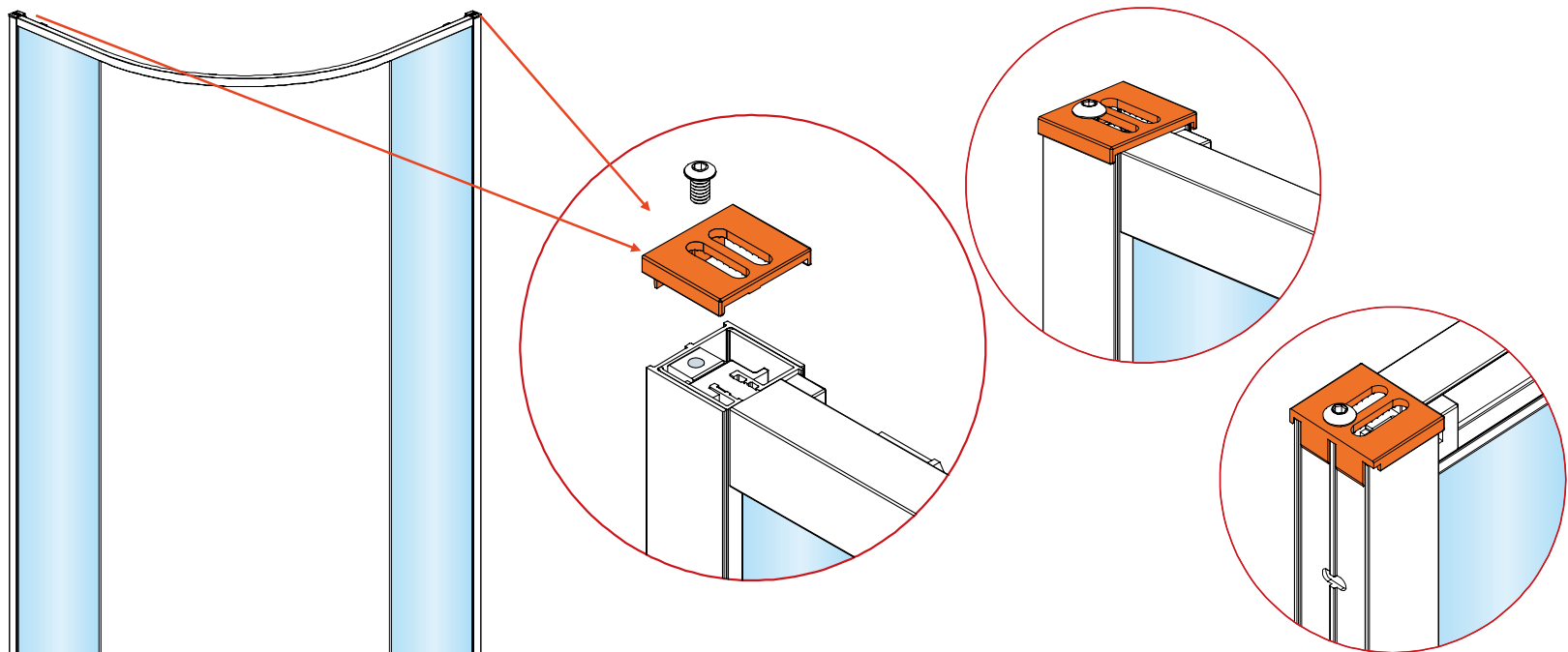
REGOLARE L'ESTENSIONE DEL PROFILO A MURO TRAMITE IL COPRIPROFILO. Wall profile and the vertical profile can be adjusted by the cover caps. Die Länge des Verlängerungsprofil durch den Profildecken feststellen. Ajuster l'extension du profilé mural par le capuchon.
