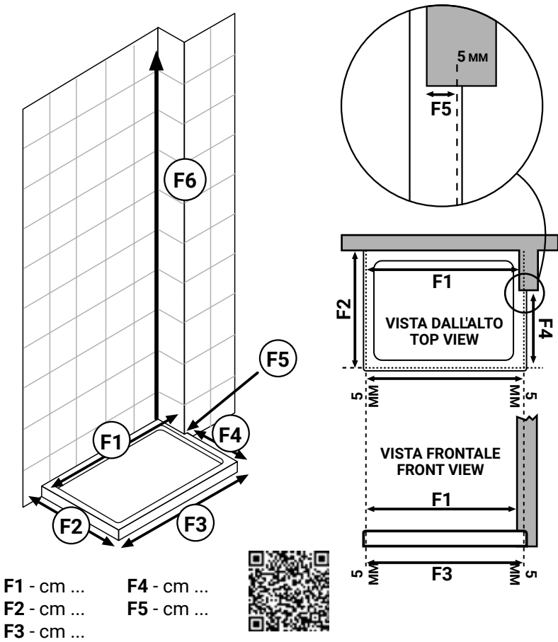
"H" - Spazio in nicchia con muretto Dx Niche with half wall on the right. - Nische mit niedriger Mauer rechts. Niche avec muret bas à droite.
