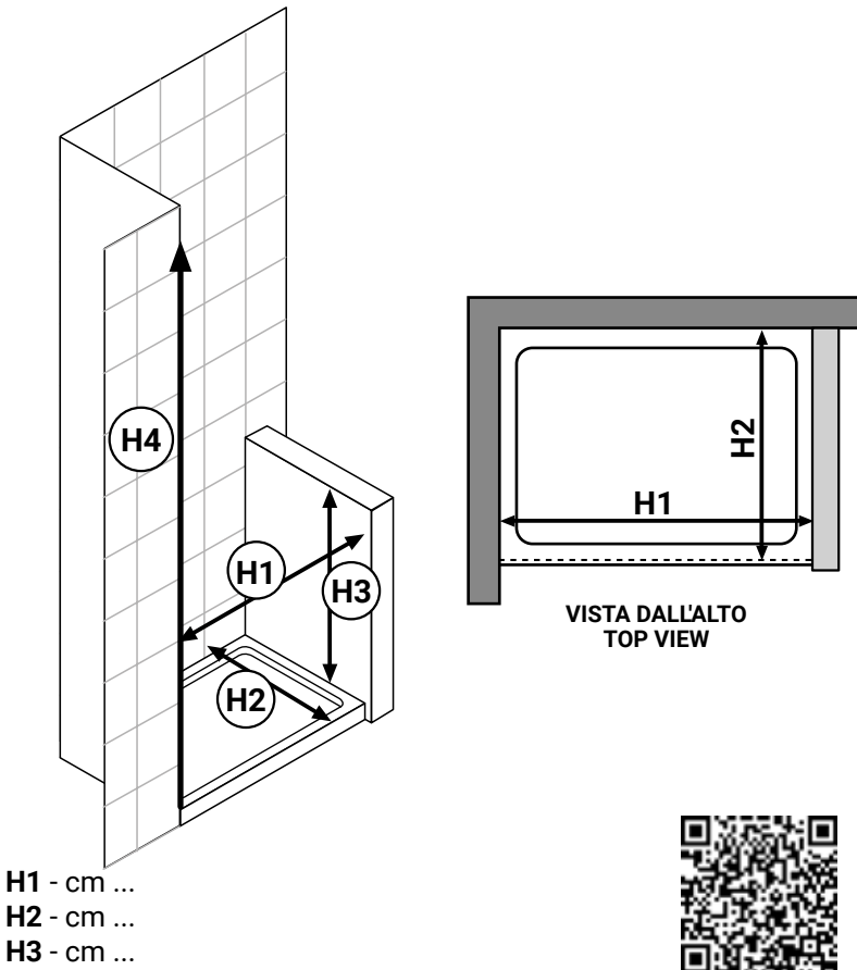
"H" - Spazio in nicchia con muretto Dx Niche with half wall on the right. - Nische mit niedriger Mauer rechts. Niche avec muret bas à droite.
